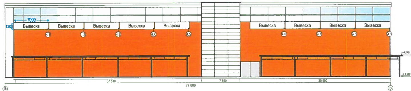
Фасад №4 в осях а - б
