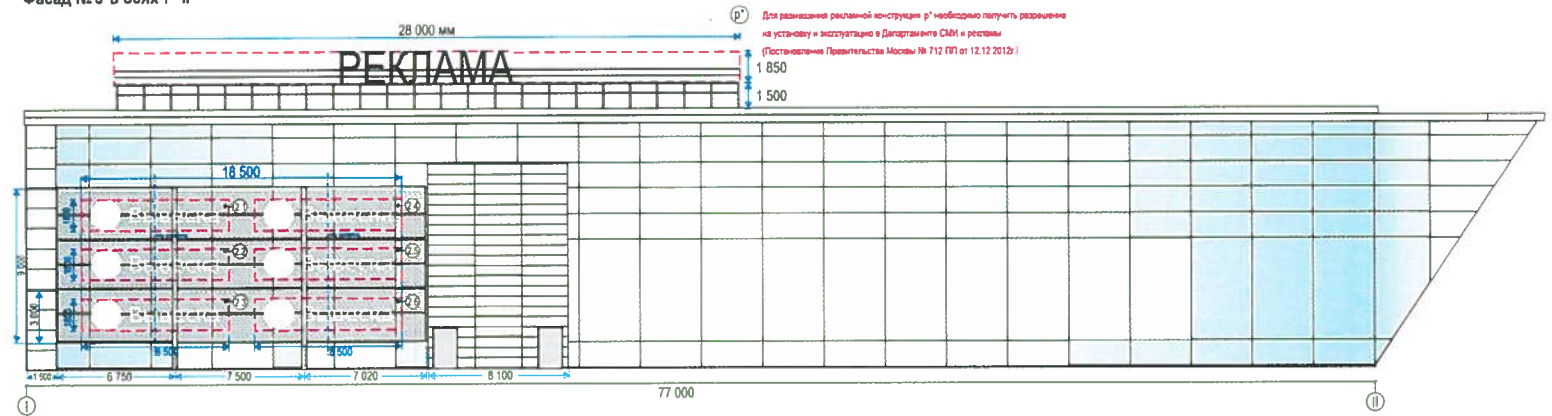
Фасад №3 в осях I - II
